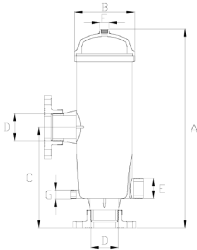
ITEM 793 | FILTRO DE MALLA SALIDA CON BRIDAS
