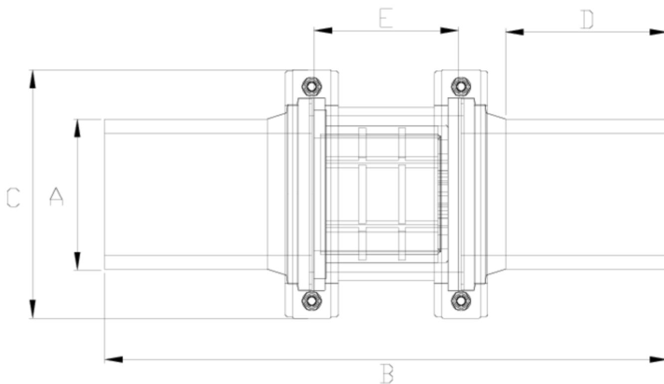
ITEM 517 | Filtro en línea salida pe-pe - visor de malla
