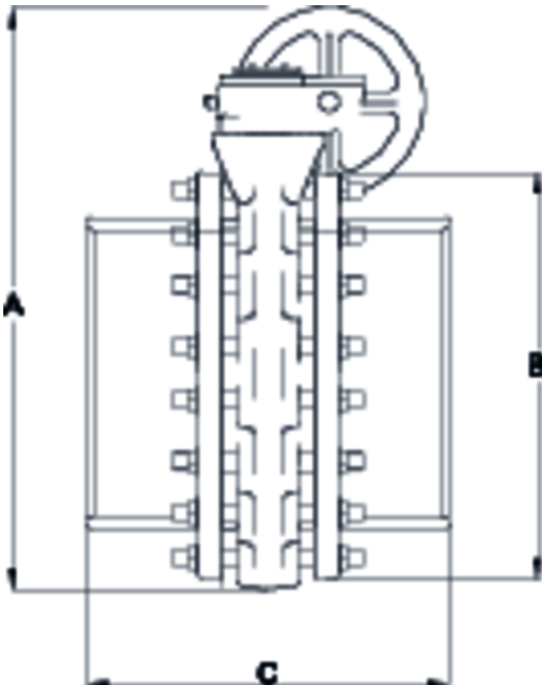
ITEM 185XXL | Válvula de borboleta Implex com redutor manual Ø400
