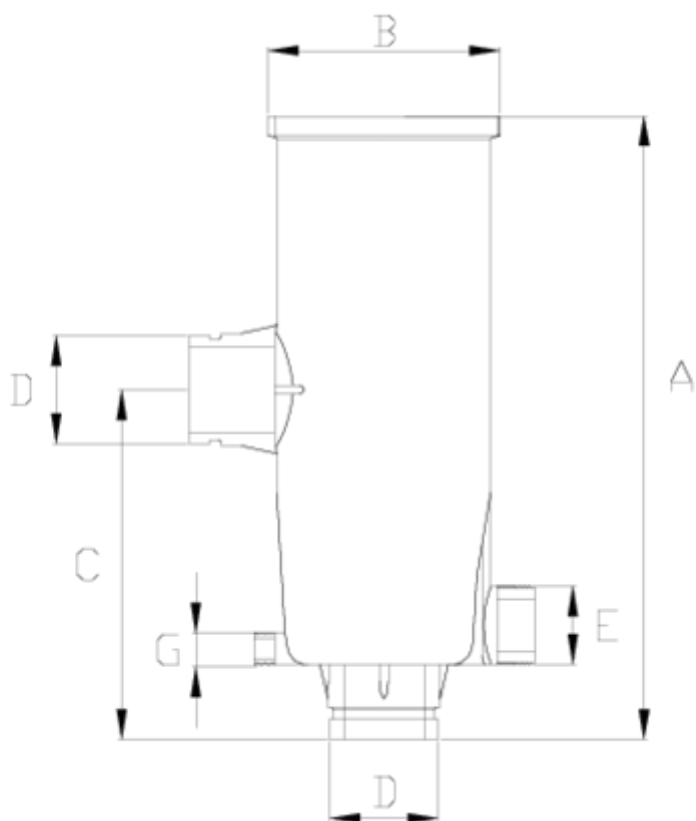
ITEM 702 | CUERPO FILTRO de anillas SALIDA NETVITC PPFV
