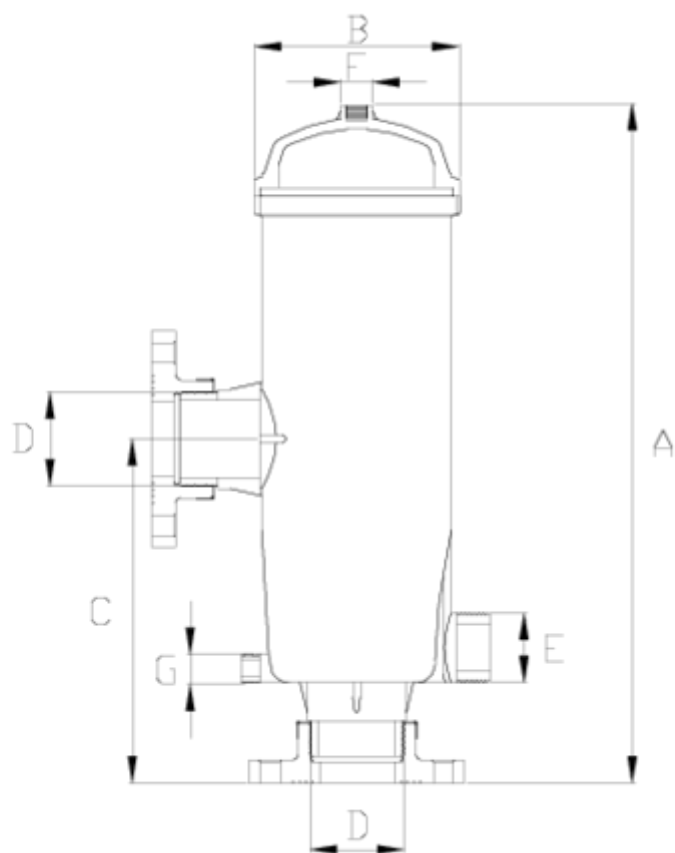
ITEM 801 | Filtro de cilindro perforado salida flanges
