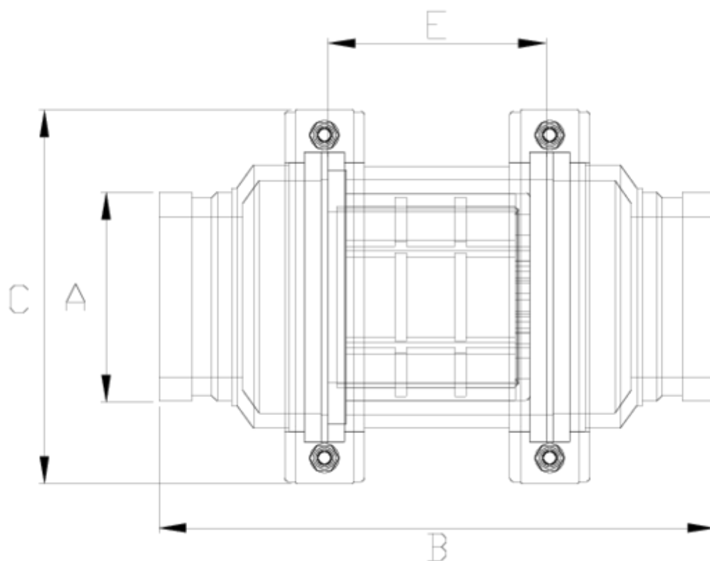
ITEM 516 | Filtro en línea salida Netvitc® - visor de malla
